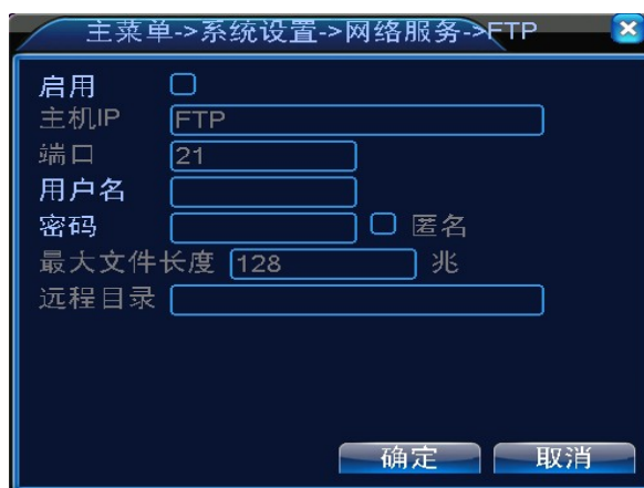
图 4.23 FTP 设置
